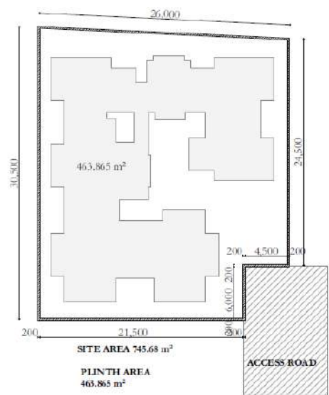
SITE PLAN 1:150
